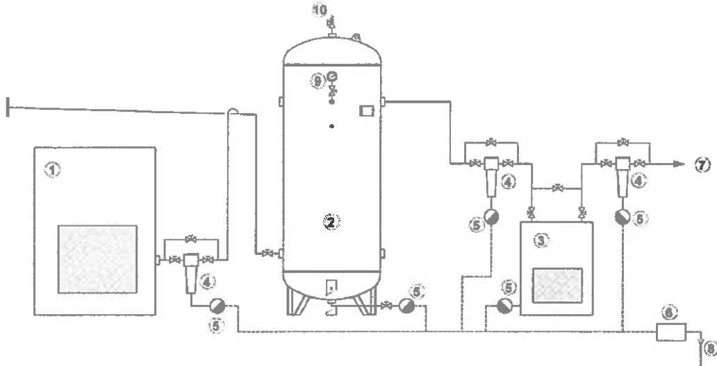
Schema impianto con serbatoio verticale
