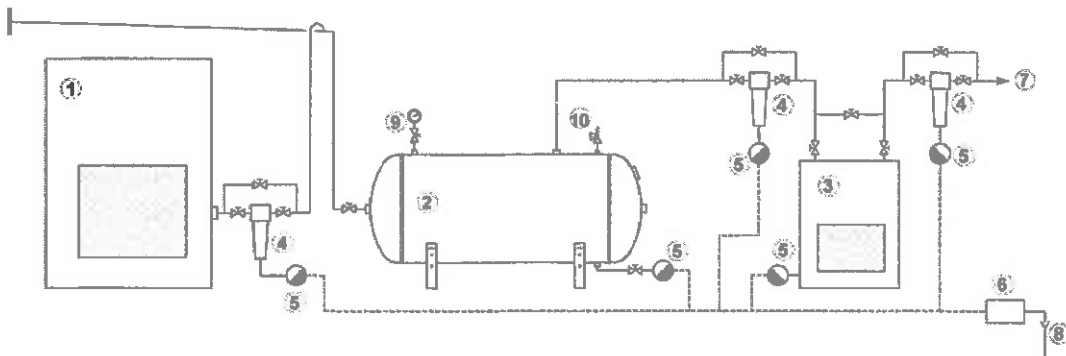
Schema impianto con serbatoio orizzontale
